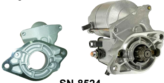
SN-8524 1.4kw, CW, 9T OEM:228000-153
